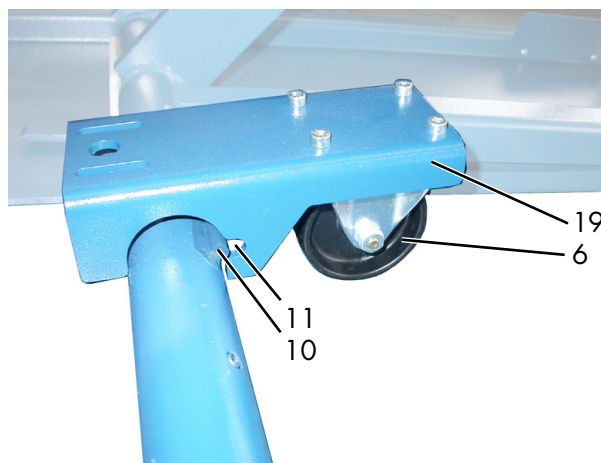
6 Rullo di rinvio 10 Trascinatore 11 Asola 19 Supporto rullo di rinvio 005
