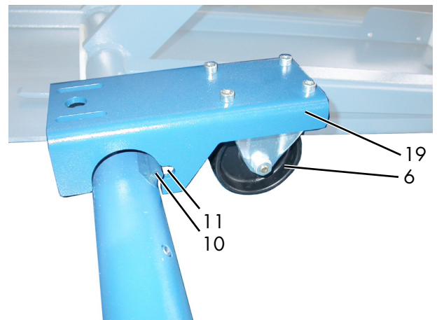
6 Lenkrolle 10 Mitnehmer 11 Ausschnitt 19 Lenkrollenhalter 005
