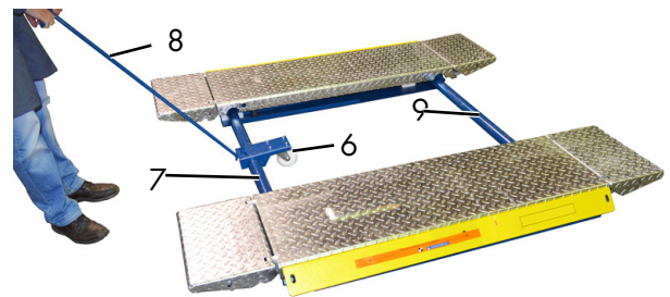
6 Lenkrolle 7 Torsionswelle 8 Deichsel 9 Radachsen Abbildung ähnlich 004
