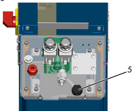
5 Apertura di riempimento olio 026
