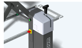
Nussbaum Commander: permite velocidades de bajada variables
